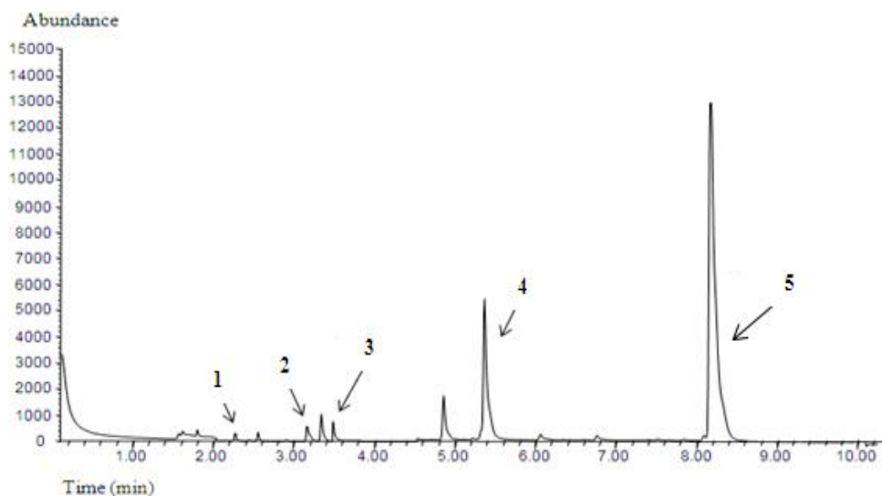
شکل 2. کروماتوگرام GC-MS ترکیبات فرار فرمولاسیون نانولیپوزمی تهیه شده به روش سونیکاسیون میله‌ای 1. پروپانال RT: 2/25، 2. پنتانال RT: 2/25، 3. استاندارد داخلی RT: 3/55، 4. هگزانال RT: 5/4، 5. هپتانال RT: 8/25
